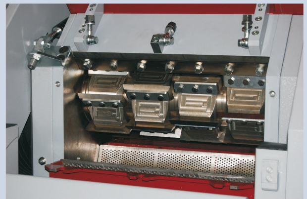
SM 1200 Schneidrotor bei geöffnetem Siebkorb
